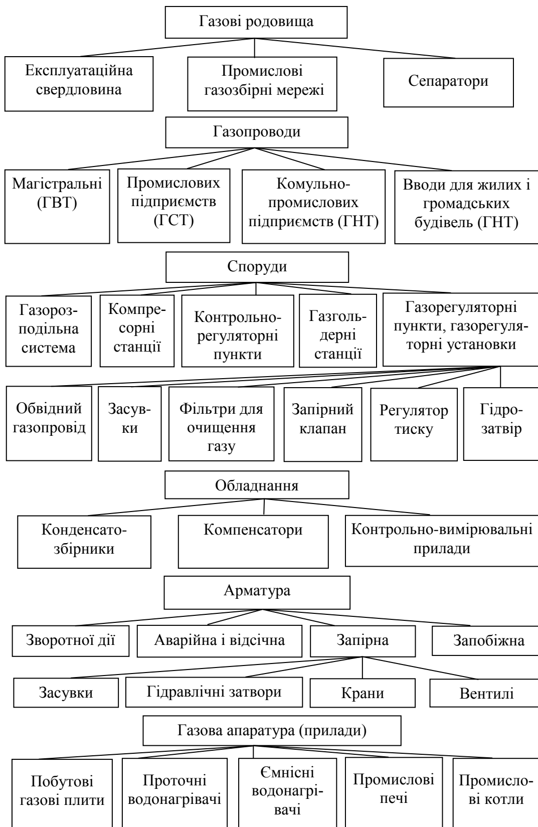
Рисунок 1.1 – Структурна схема системи газопостачання
