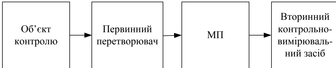
Рисунок 1.2 – Усічена структурна схема засобу контролю активності іонів
