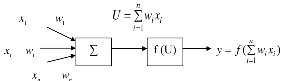
Рис. 1.2. Модель штучного нейрона
