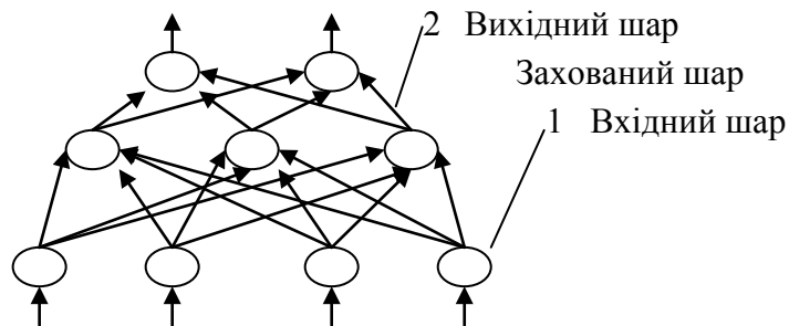
Рис. 1. 3. Структура нейронної мережі: 1 – нейрон; 2 – зважений зв'язок
