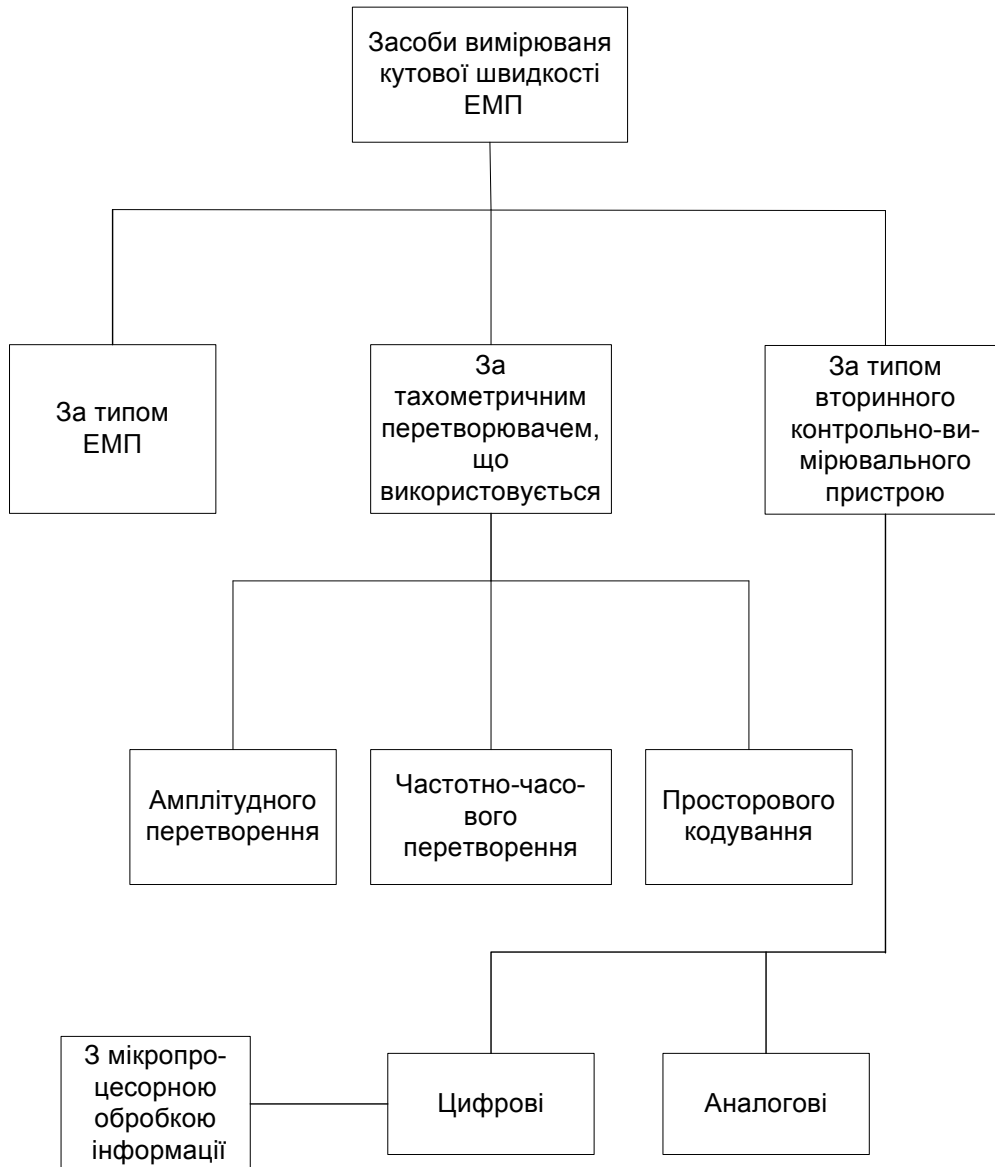
Рис.1.5. Класифікація засобів вимірювання кутової швидкості ЕМ
