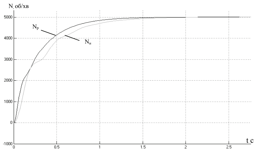
Рис. 1.2. Перехідні характеристики регульованого і нерегульованого ЕМ
