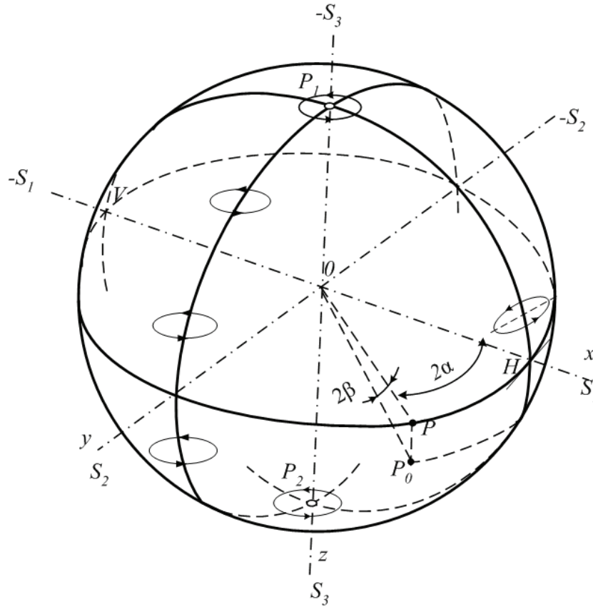
Рис. 1.3. Сфера Пуанкаре станів поляризації
