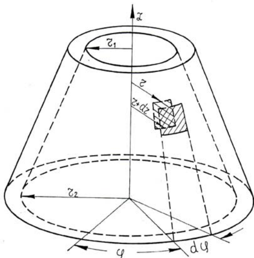
Рисунок 1.4 – Шар газу між співвісними конічними поверхнями
