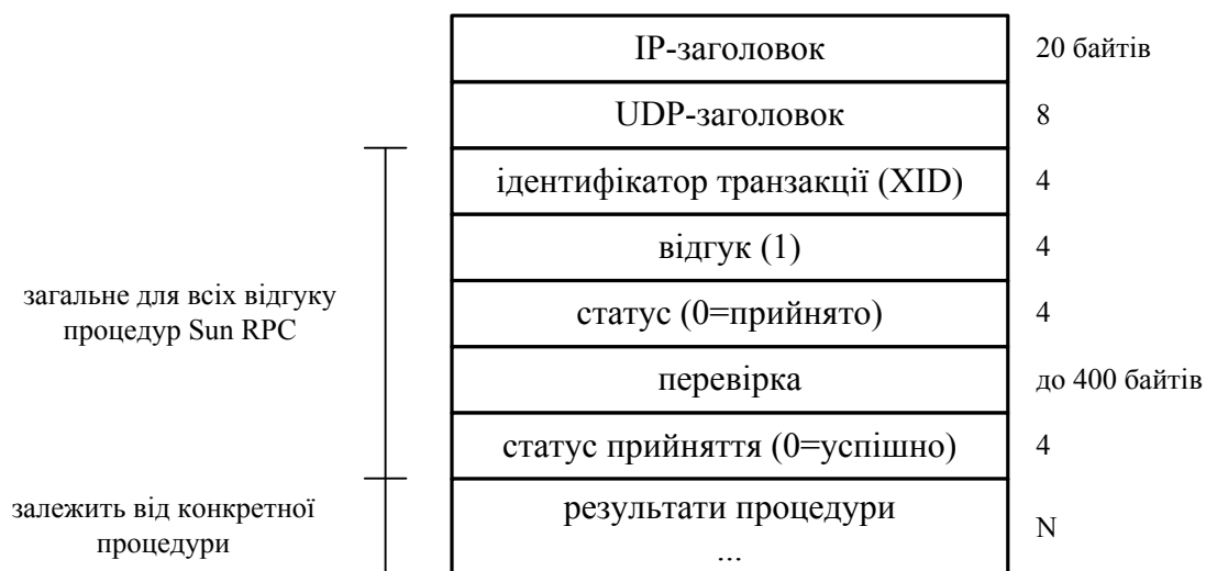
Рисунок 6.16 – Формат відгуку процедури RPC у форматі UDP-дейтаграми
