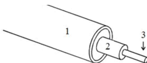
Рисунок 2.8 – Структура оптоволоконного кабелю
