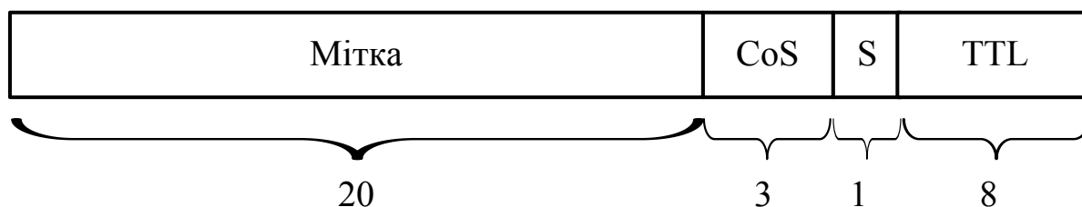
Рисунок 8.20 – Формат заголовка MPLS
