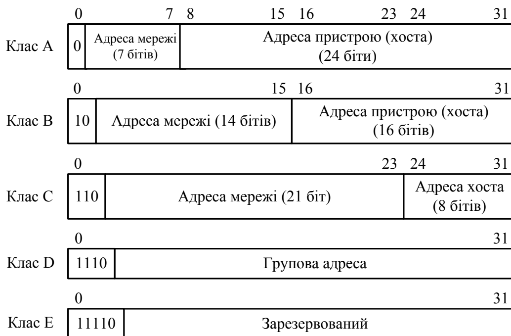
Рисунок 4.1 – Структури IP-адрес різних класів
