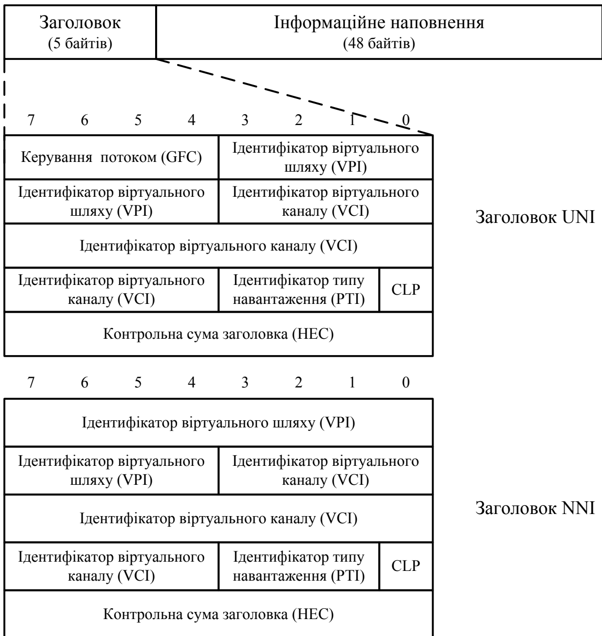
Рисунок 8.16 – Структура комірки АТМ
