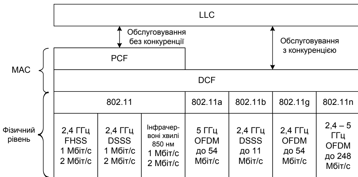
Рисунок 9.6 – Стек протоколів IEEE 802.11
