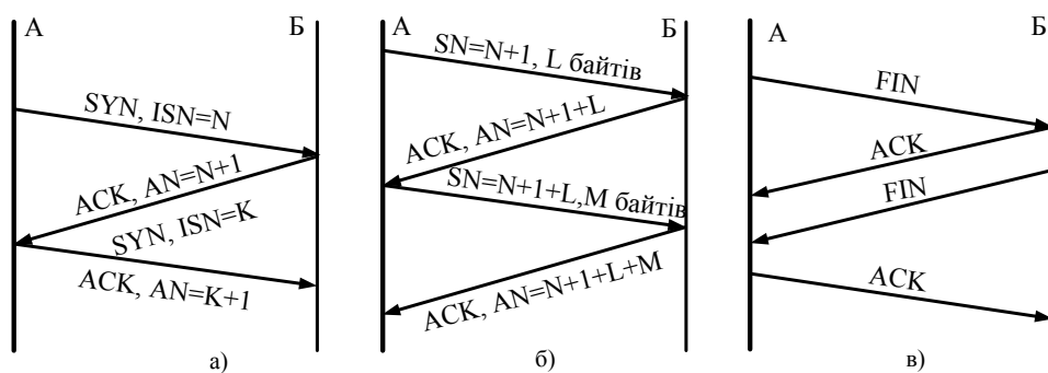
Рисунок 5.5 – Робота протоколу ТСР
