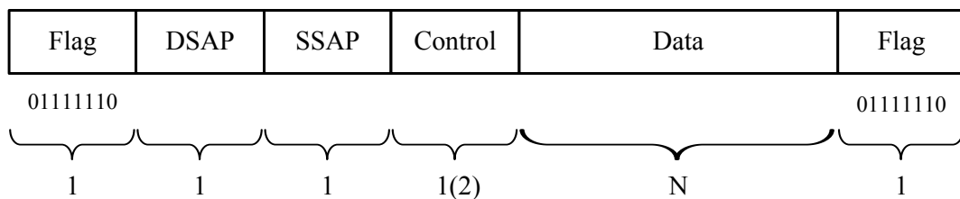
Рисунок 3.12 – Формат кадру LLC
