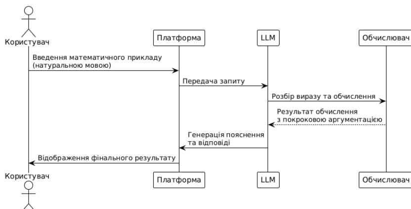
Рис. 1. UML-діаграма послідовностей інтеграції дистильованої великої мовної моделі (LLM) для автоматичного обчислення математичних завдань
