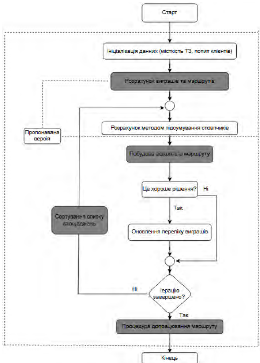
Рисунок 1.1 – Алгоритм роботи методу Кларка-Райта.
