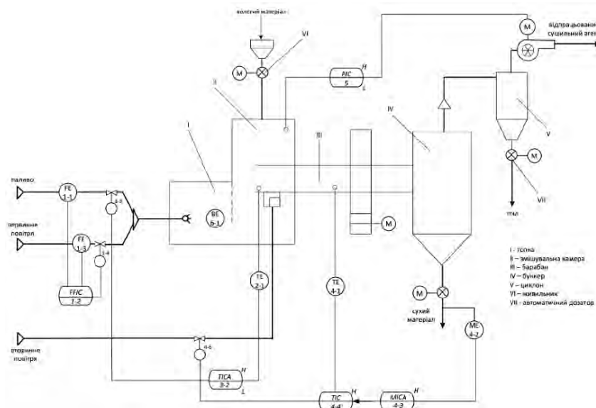
Рисунок 4 — Спрощена функціональна схема автоматизації (ФСА) процесу сушіння глини в проточній барабанній сушарці
