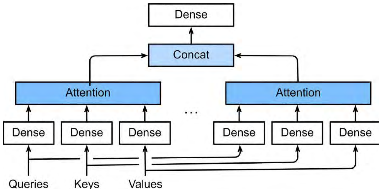
Рис. 2. Ілюстрація концепції блоку з багатоголовою увагою
