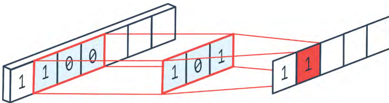
Рис. 3. Принцип роботи одновимірного фільтра згорткового шару
