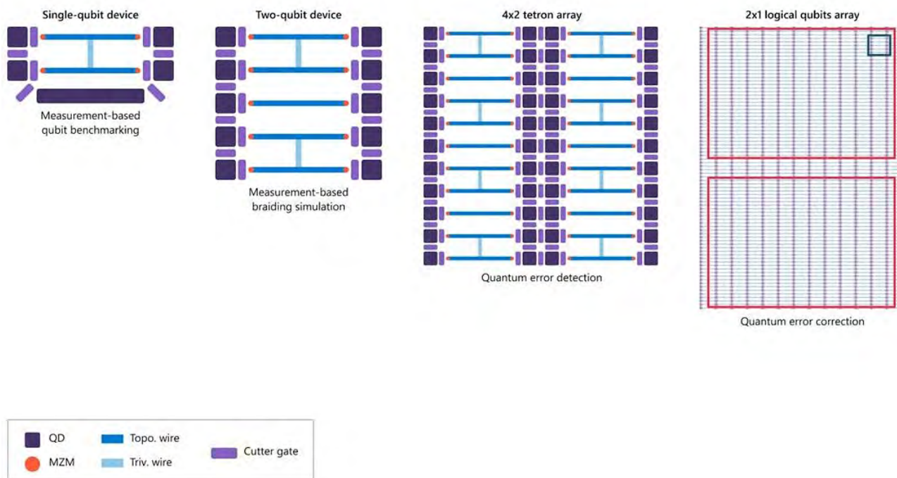
Рис. 2 Масштабування топологічних квантових пристроїв для корекції помилок
