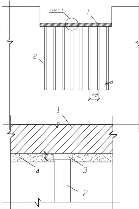
Рис. 1 Плитно – паливовий фундамент
