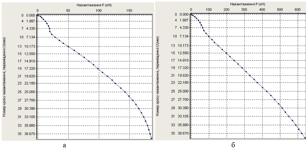
Рис. 2 – Графік «навантаження – осідання» результатів розрахунку за МГЕ, а) фундаменту без підсилення, б) підсиленого буроін'єкційними палями за числовим МГЕ
