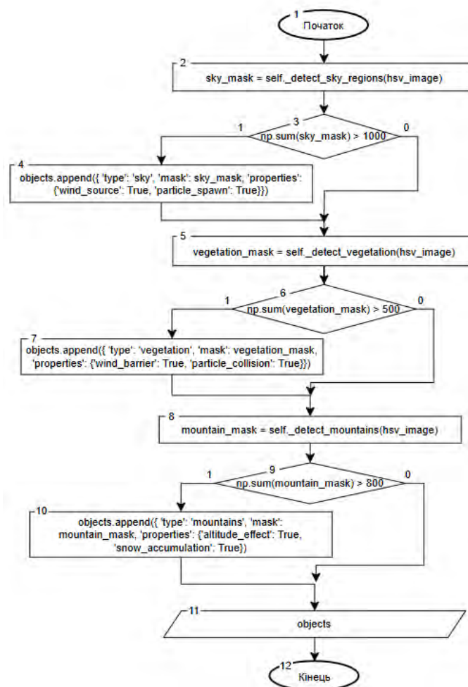
Рисунок 3 - Блок-схема алгоритму детекції об'єктів сцени
