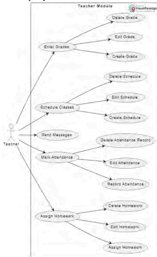
Рисунок 1.1 - Use Case UML-діаграма модуля користувача в ролі Вчитель
