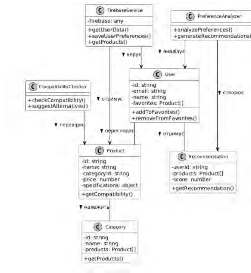
Рисунок 3 – Діаграма класів веб-застосунку
