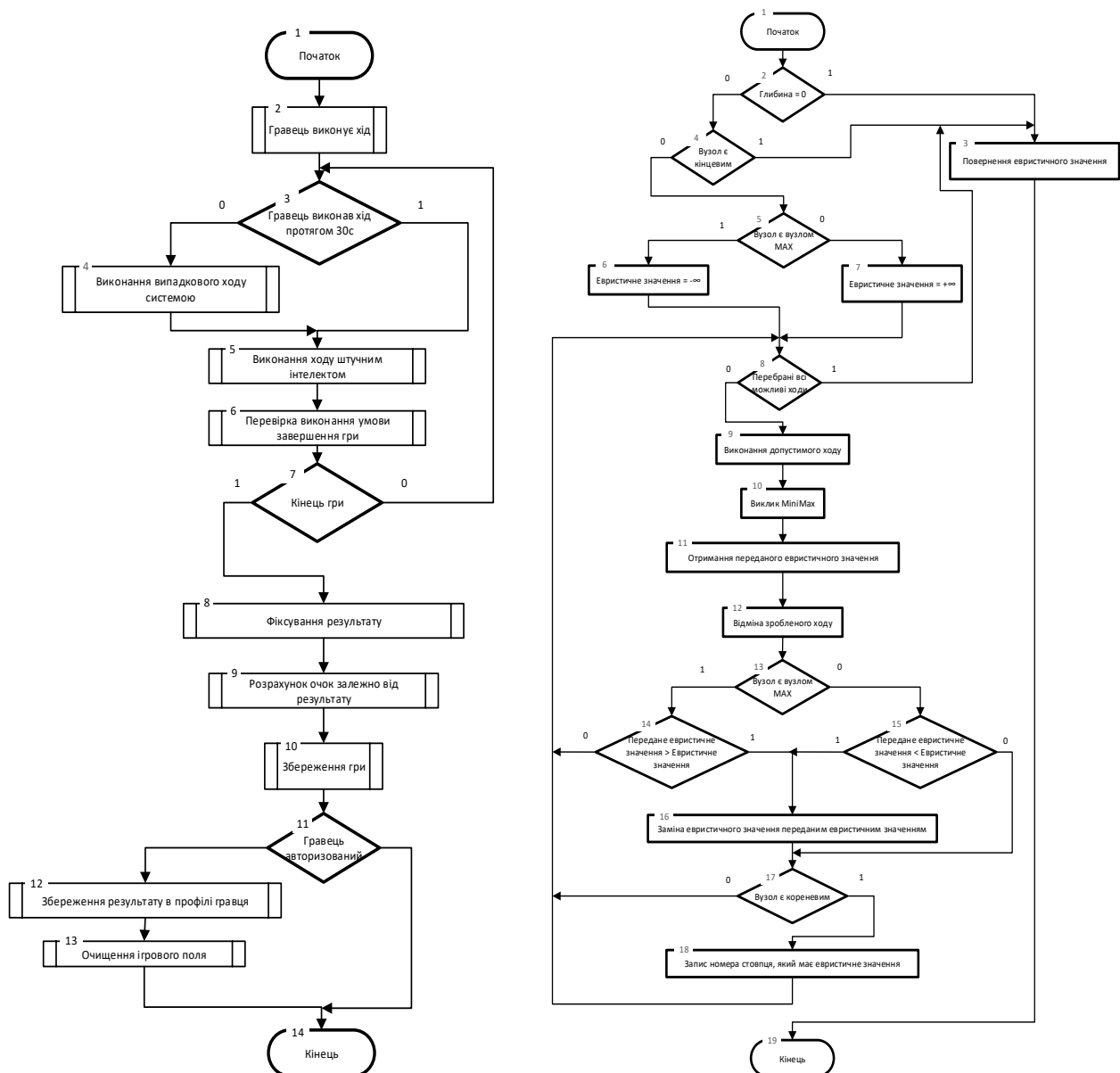
Рисунок 1 – Розроблений ігровий алгоритм MiniMax. а) Алгоритм гри проти штучного інтелекту б) Алгоритм MiniMax роботи штучного інтелекту
