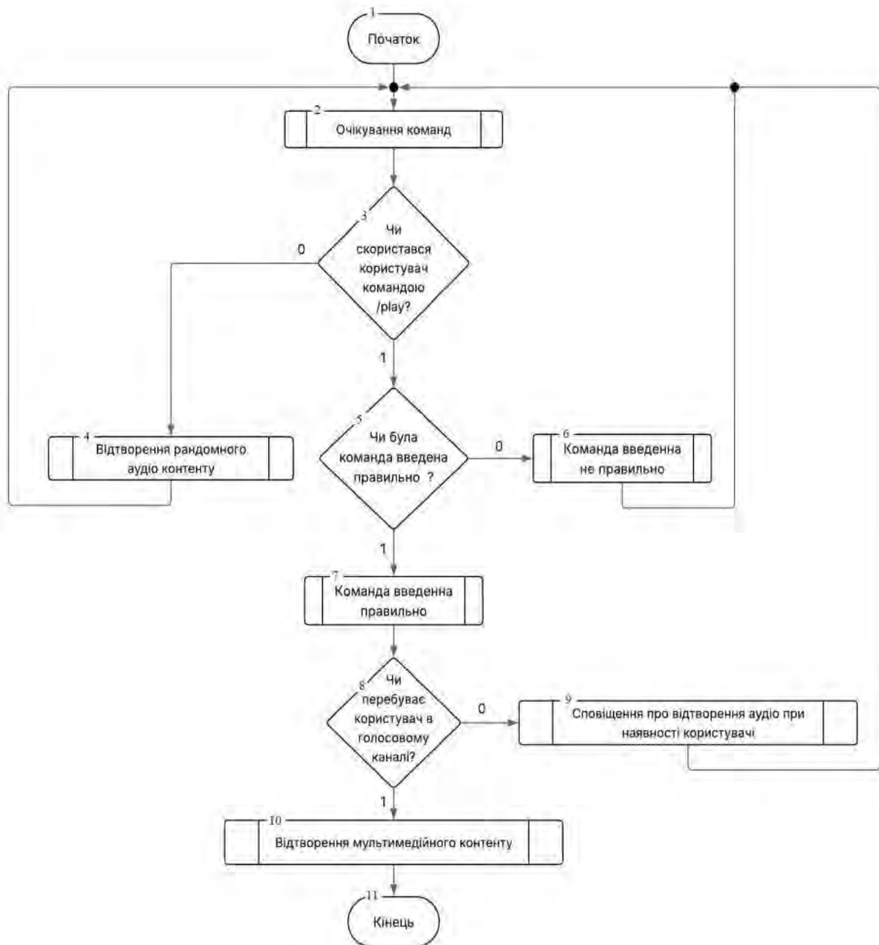
Рисунок 2 – Блок-схема алгоритму реалізації динамічного пошуку та керування відтворенням аудіоконтенту
