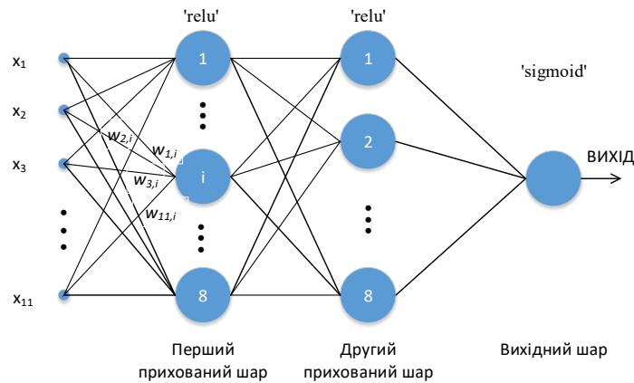
Рисунок 1 – Структура багатошарового персептрона для інформаційної технології визначення якості вина
