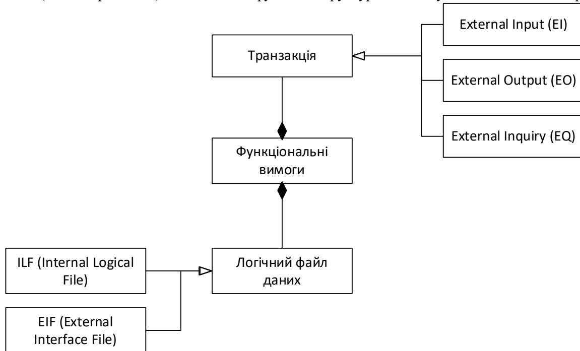
Рис. 1. Модель сутностей FPA за IFPUG
