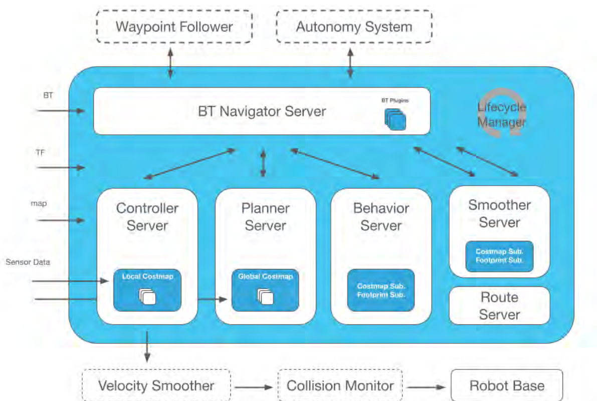
Рисунок 1 – Архітектура роботи nav2 з офіційної документації
