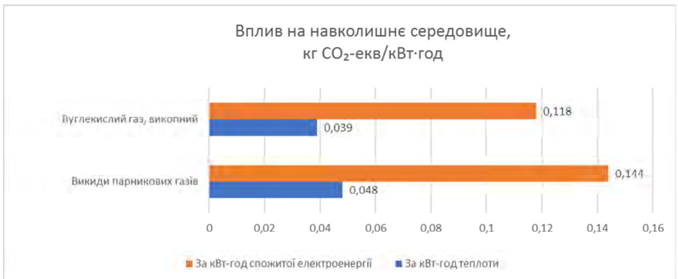
Рис. 5 – Результати моделювання екологічних показників в «Калькуляторі теплового насосу»
