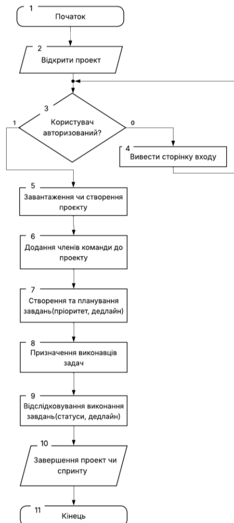
Рисунок 1 – Загальний алгоритм роботи вебсистеми
