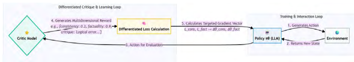
Рисунок 1 – Тренувальний цикл запропонованого підходу
