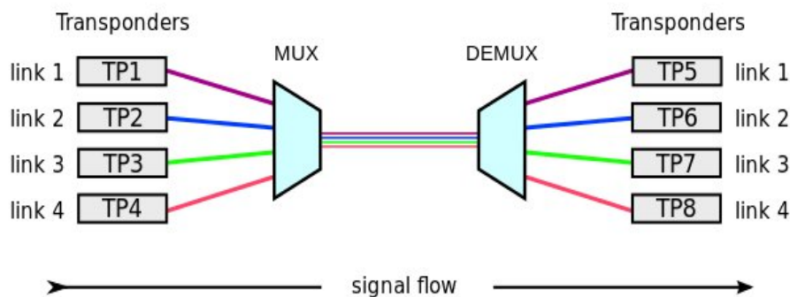
Рис.2 – Спрощена схема WDM
