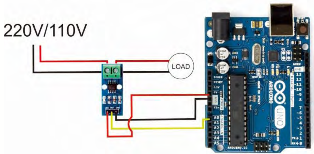
Рисунок 1 - Схема пристрою
