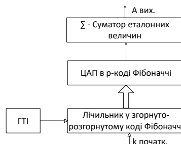
Рисунок 3 – Низькогітчевий ЦАП на основі згорнуто-розгорнутих кодів Фібоначчі
