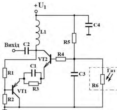
Рис. 1. Еквівалентна схема параметричного автогенераторного сенсора концентрації газу
