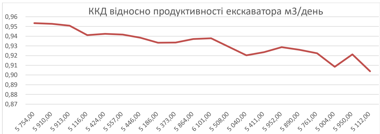
Рисунок 2 – ККД екскаватора відносно фактичної продуктивності екскаватора \text{м}^3/\text{день} для плаstopодібної породи
