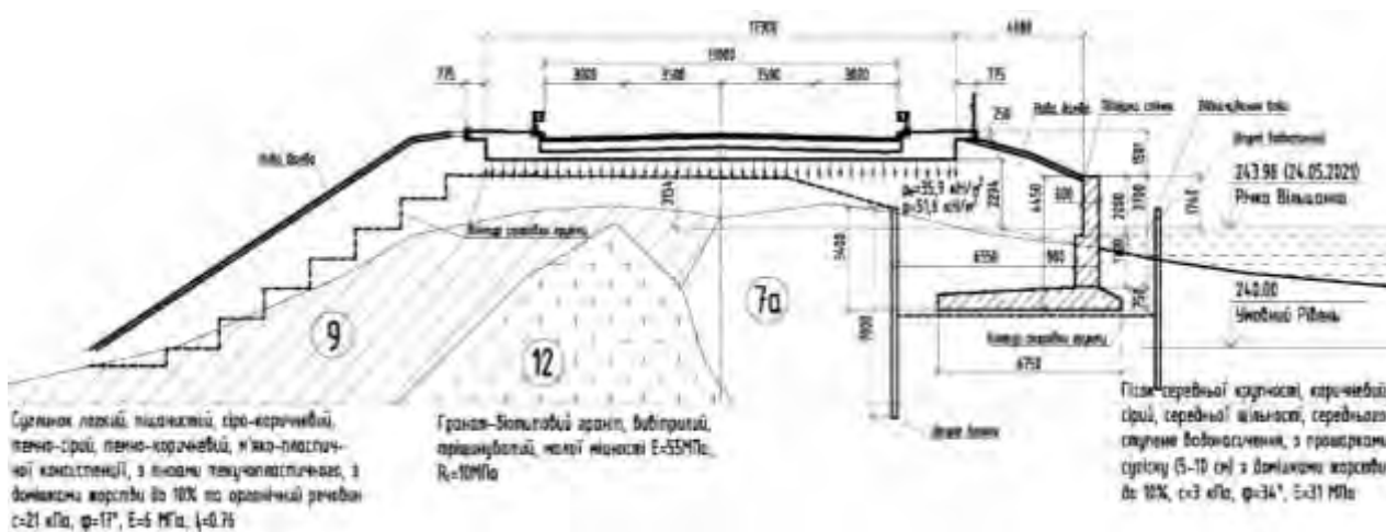
Рис. 1. Конструктивна схема улаштування берегоукріплення проектового підходу мостового переходу через р. Вільшанка у селищі Турбів у вигляді кутикової підпірної стінки у місці улаштування перехідних конструкцій.
