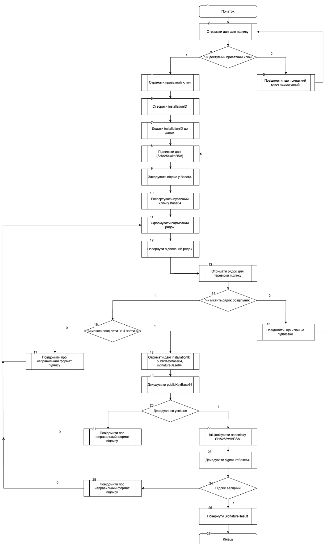
Рисунок 1 – Алгоритм роботи цифрового підпису
