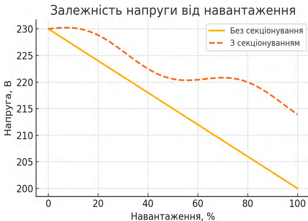
Рис. 1 — Залежність напруги від навантаження при різних режимах
