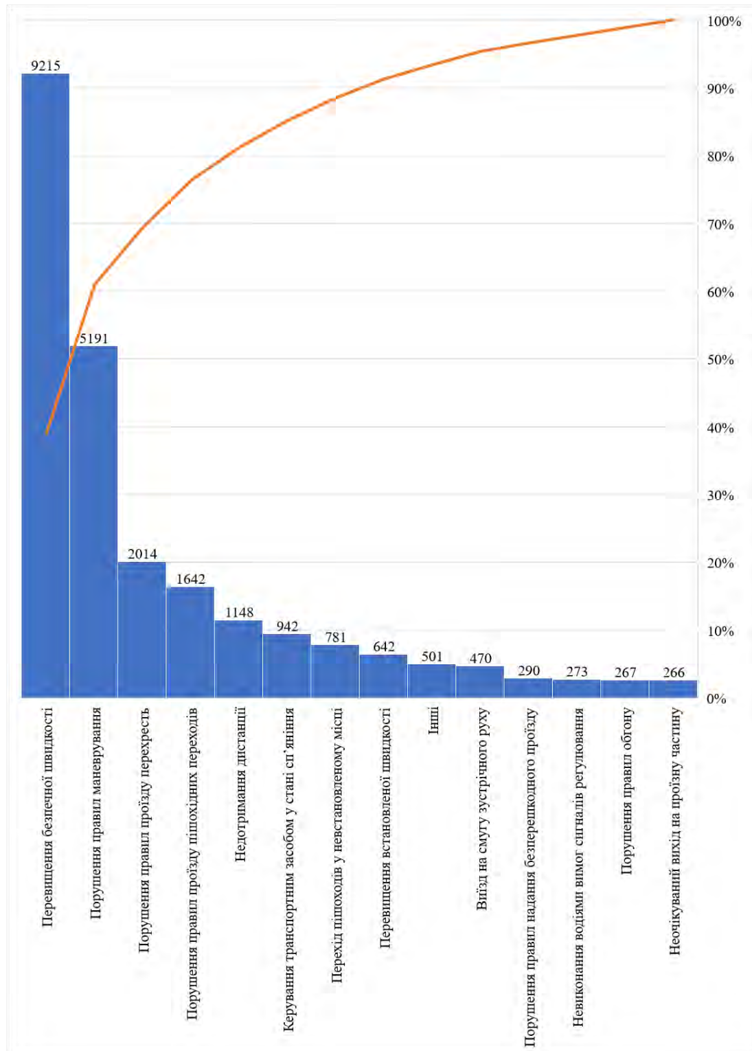
Рисунок 2 – Причини аварійності 1-ї групи
