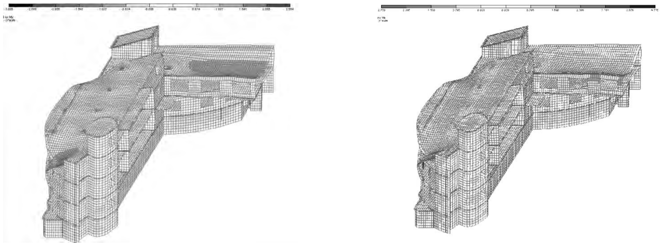
Рисунок 2 – Ізополю внутрішніх зусиль скінченно-елементної моделі 3-поверхової будівлі з підвалом а) M_x , б) M_y
