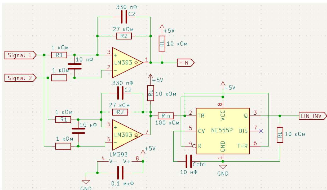
Рис. 2. Принципова схема гістерезисного методу керування
