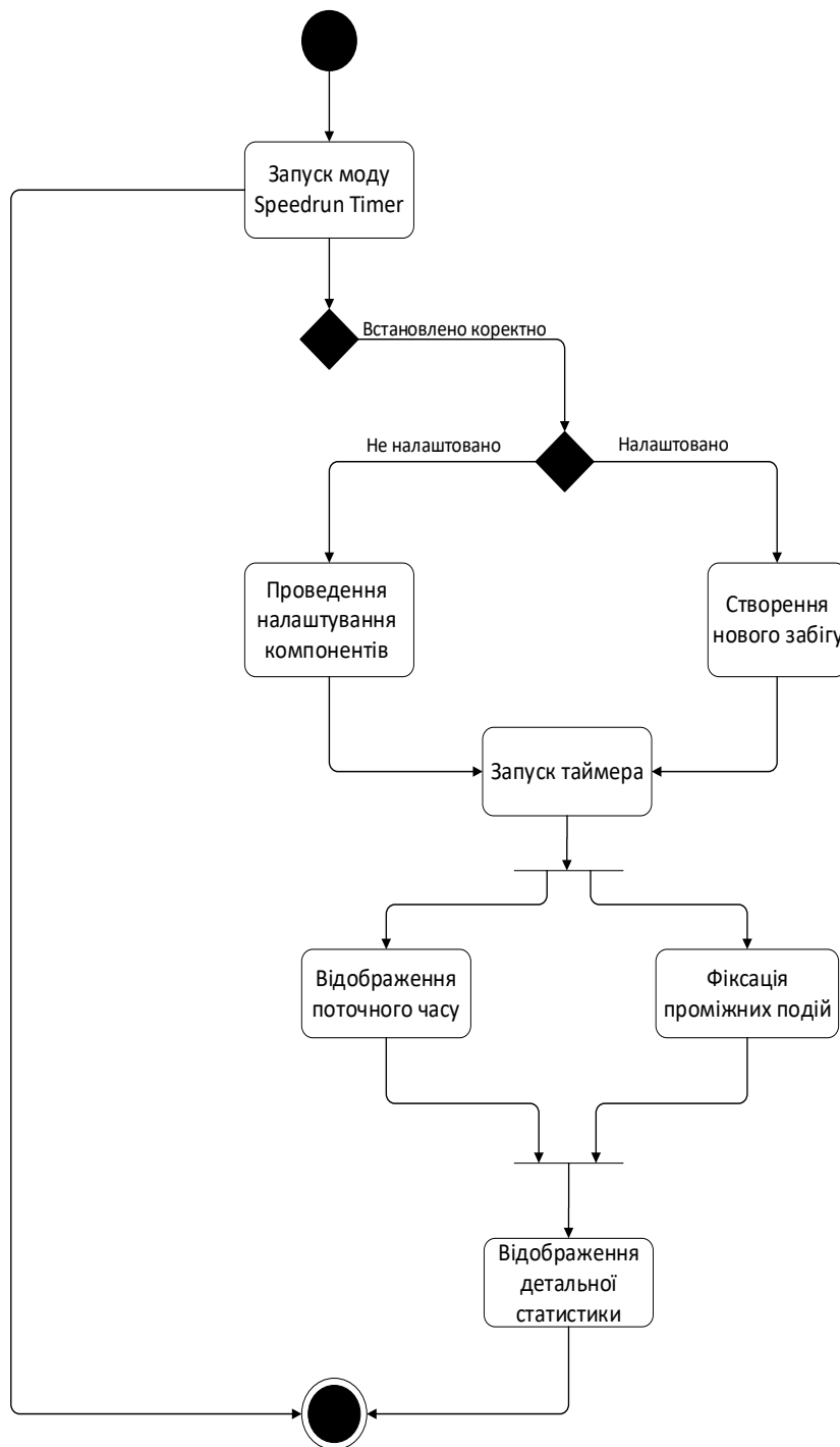
Рис. 2. Діаграма станів модуля відслідковування ігрових подій
