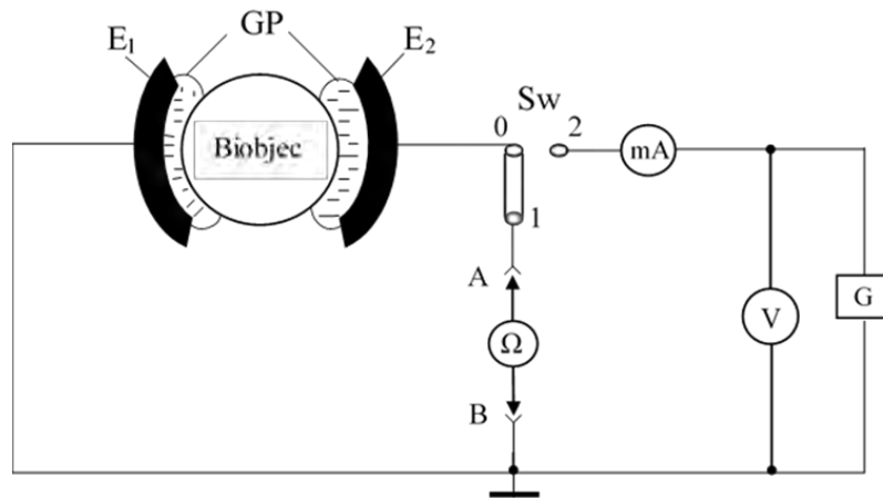
Рисунок 1 – Електрична схема дослідження
