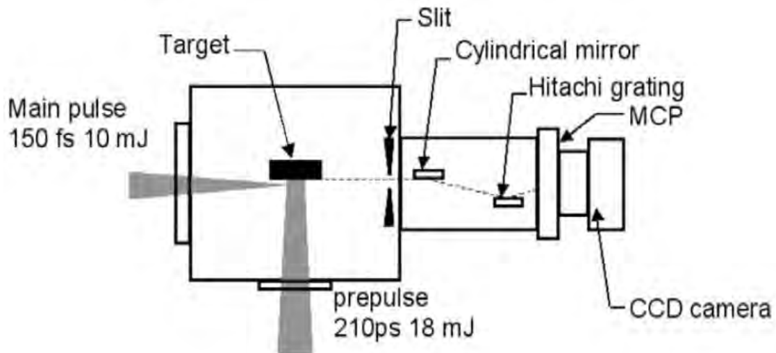
Установка HHG
