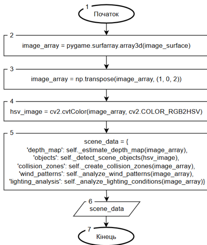
Рисунок 1 — Блок-схема алгоритму інтелектуального аналізу сцени
