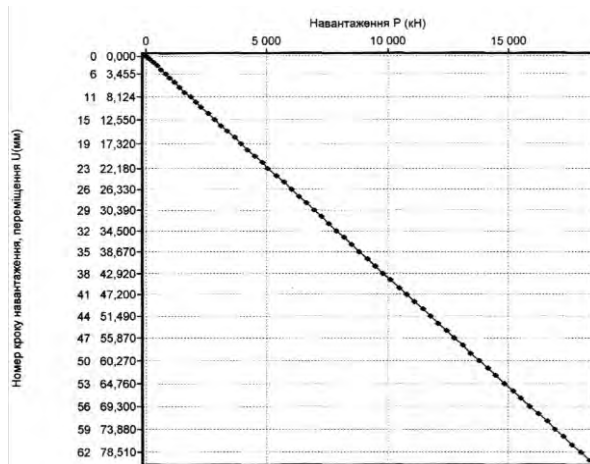
Рисунок 6 – Графік навантаження–осідання будівлі на фундаментній плиті h=50 см при заміні 1м ґрунту мілким піском, з середньозваженими характеристиками: E=17525 кПа; \nu=0,3 ; \rho=1,809 ; \varphi=0,3873 радіан; C=12,06 кПа. Вага будівлі – 18205 кПа.
