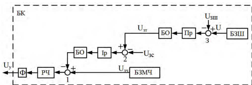
Рис. 2. Структурна схема блоку керування електропривода
