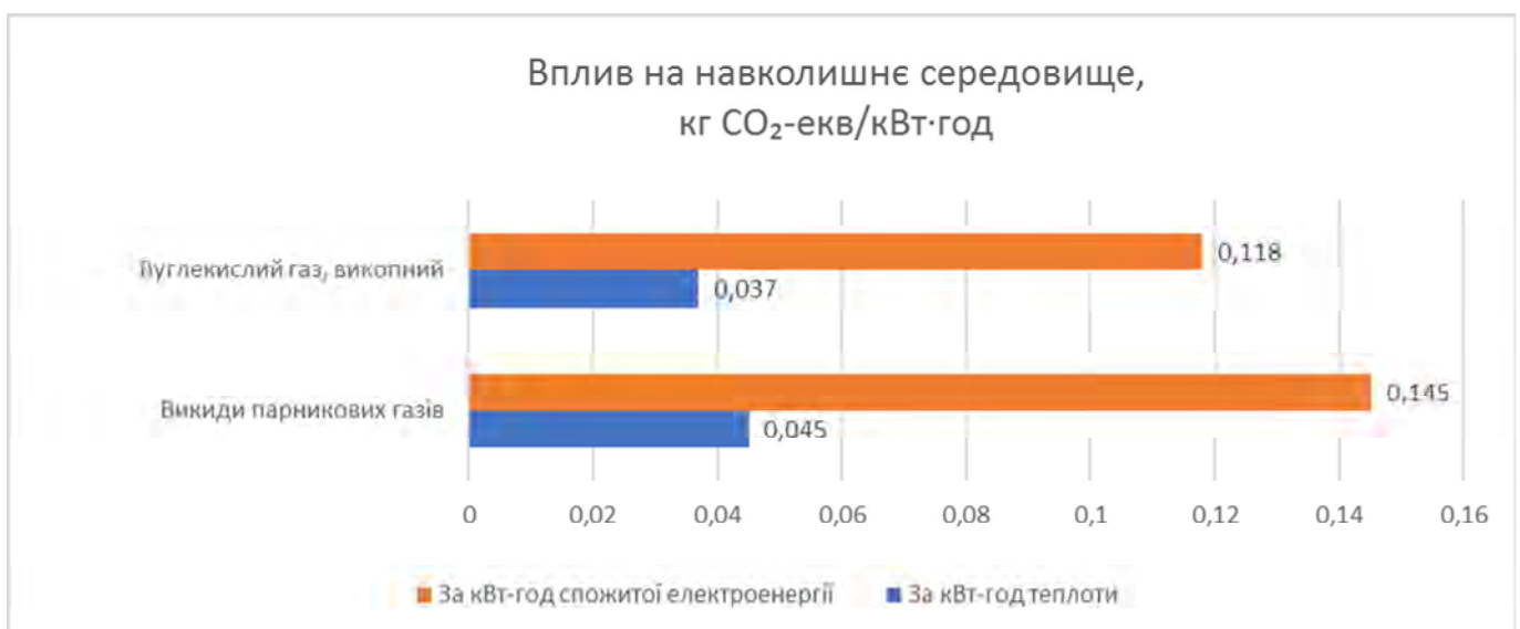
Рис. 2 – Результати моделювання екологічних показників в «Калькуляторі теплового насосу»
