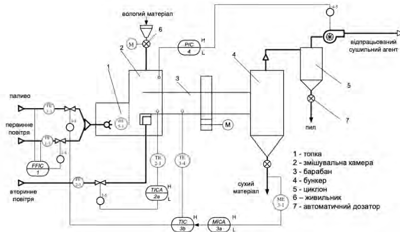
Рисунок 2 — Спрощена схема барабанної проточної сушарки
