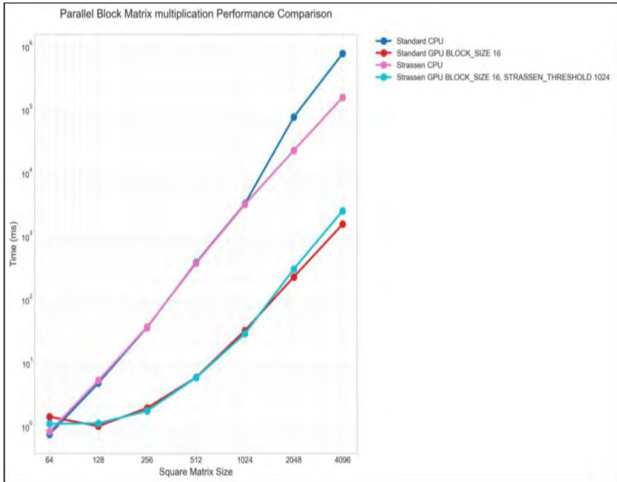
Рисунок 1 – Порівняння часу множення матриць на CPU та GPU
