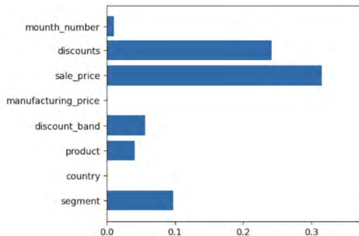
Рис. 4. Ваги властивостей у прогнозі моделі
