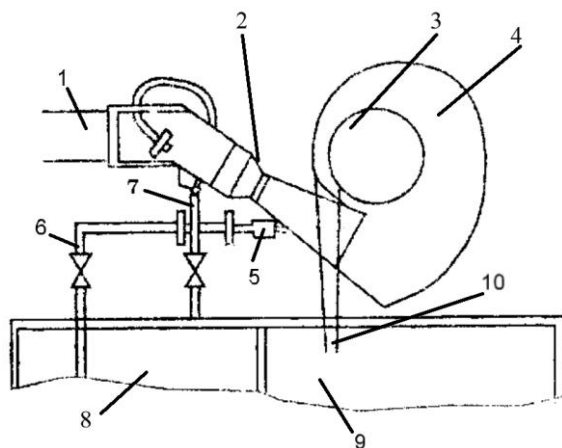
Рис. 3. Натрубний мокрий пиловловлювач: 1 - димосмок; 2 - скуббер Вентурі; 3 - димова труба; 4 — равлик відцентрового бризкоуловлювача; 5 - насосний агрегат шламовий; 6 - трубопровід всмоктуючий; 7 - трубопровід циркуляції води; 8 - блок освітленого шламу; 9 - шламовловлювач; 10 - рукав шламоуловлювача
