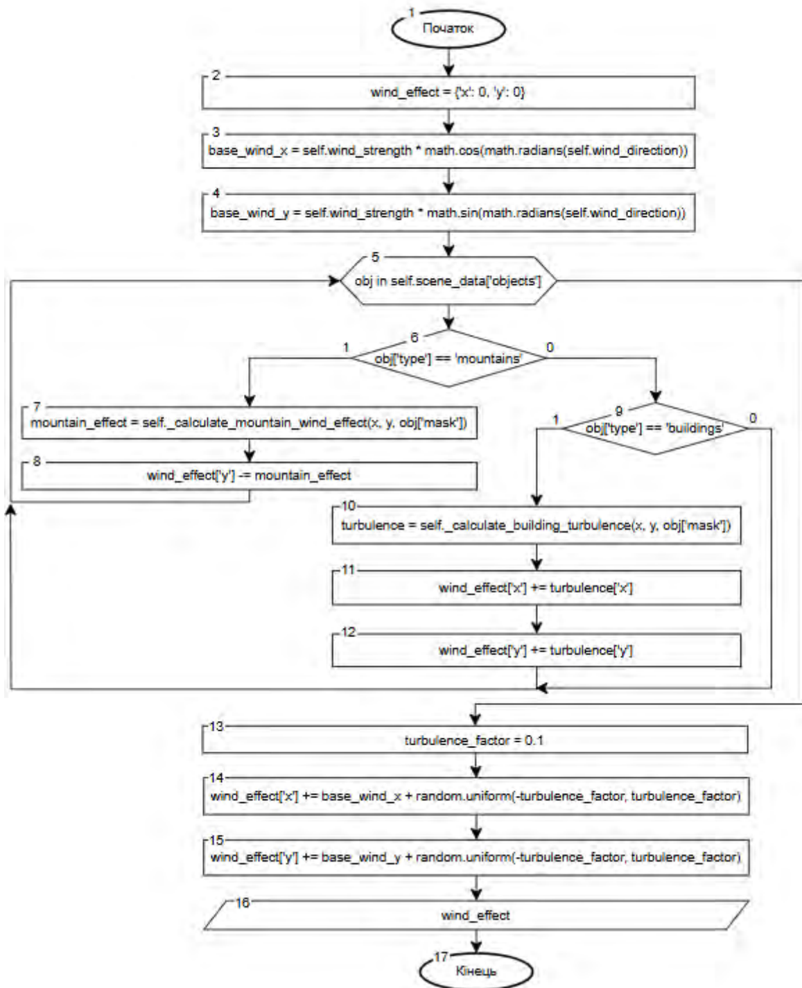
Рисунок 5 - Алгоритм розрахунку вітрового впливу
