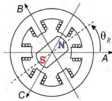
Рис. 1. Розріз двополусної безконтактної машини постійного струму
