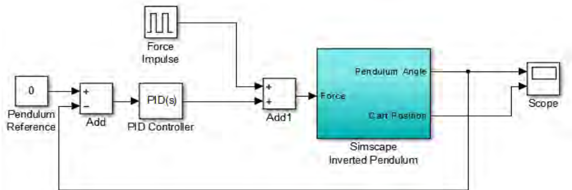
рис.1. Схема системи управління в середовищі Simulink /MATLAB
