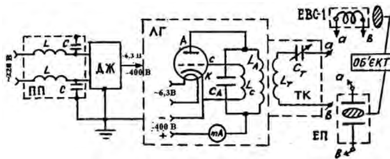
Рисунок 1.1 – Спрощена схема апарату УВЧ-30
