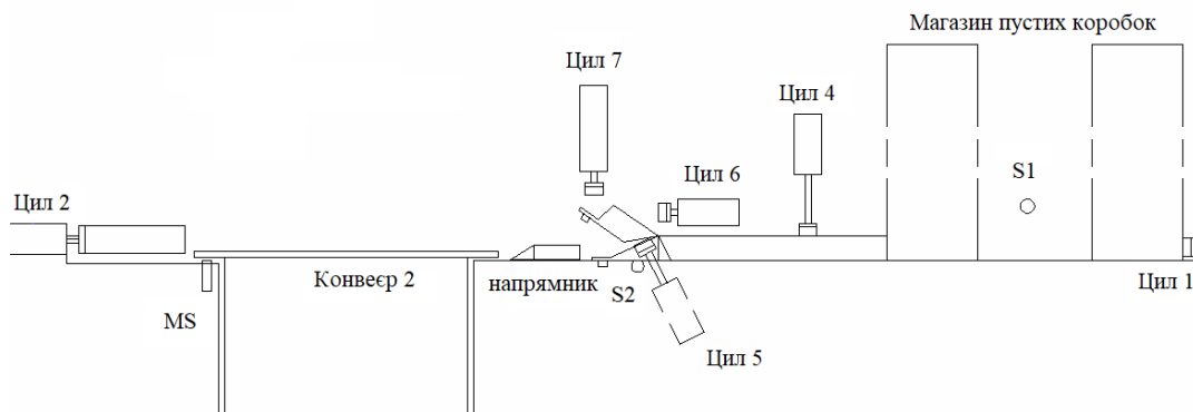
Рисунок 3 – Принципова схема пакувальної станції
