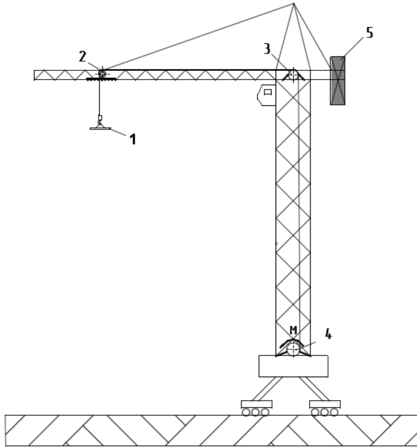
Рис.1. Конструктивна схема баштового крана
