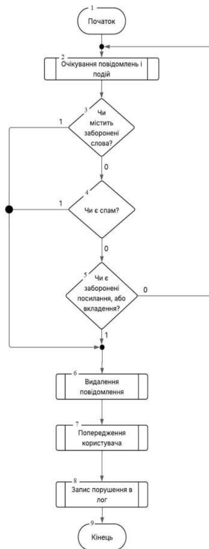
Рисунок 3 – Блок-схема алгоритму модерації контенту
