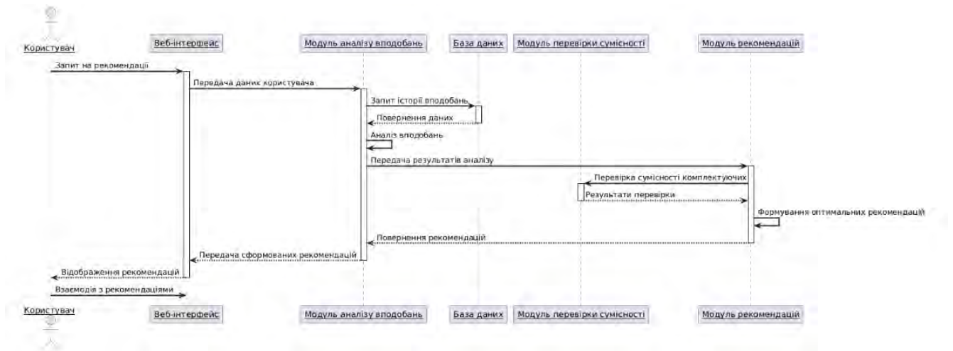
Рисунок 2 – Діаграма послідовності процесу формування рекомендацій
