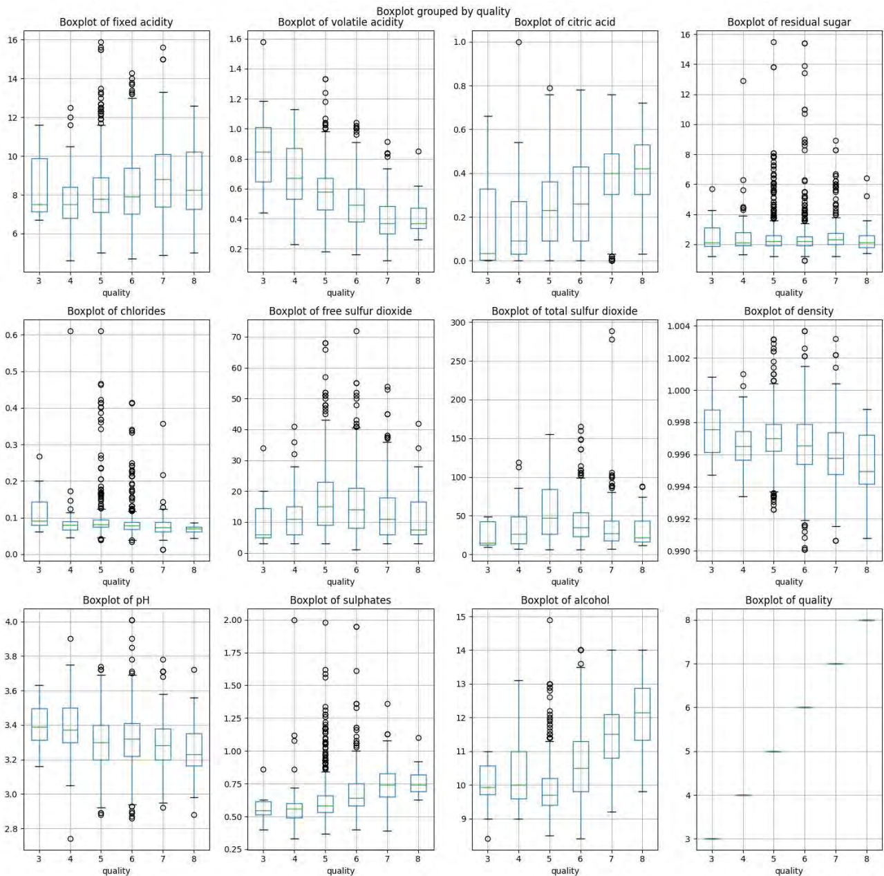
Рисунок 7 – Коробкові графі чисельних змінних з поділом на категорії цільової змінної
