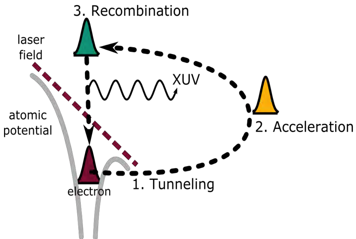
Схема трьохступеневої моделі HHG
