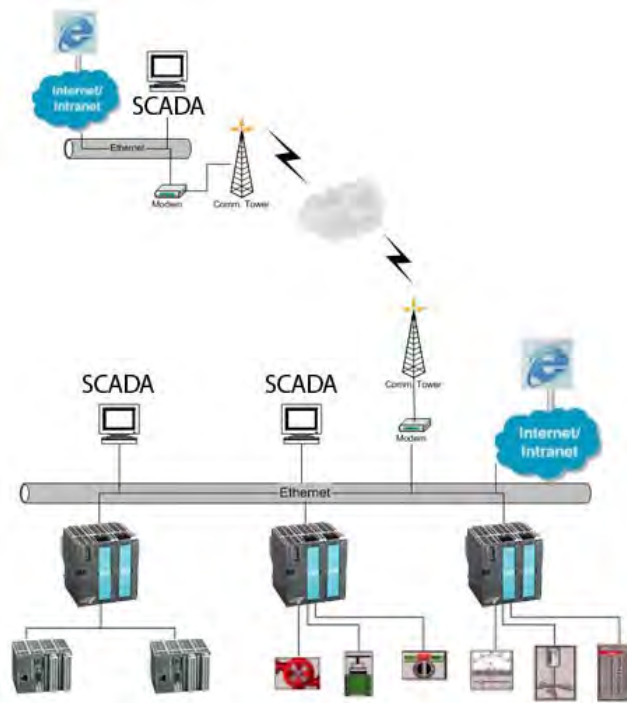
Рис. 1. Структуру SCADA-системи для управління розподіленими системами водопостачання
