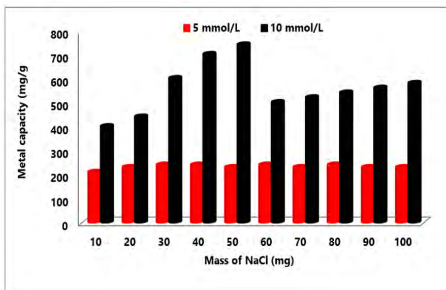
Рисунок 1 – Вплив іонної сили на здатність до видалення ртуті (мг/г) за допомогою наносорбенту
