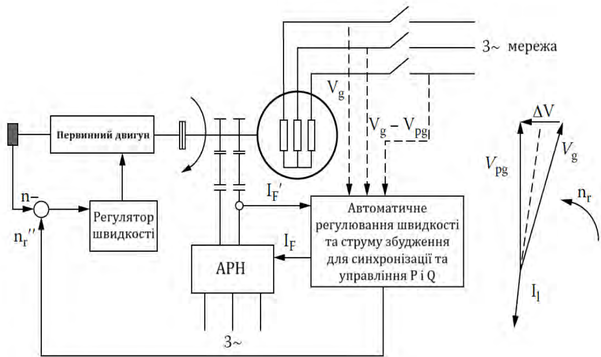
Рис. 1. Підключення синхронного генератора до енергосистеми (структурна схема)
