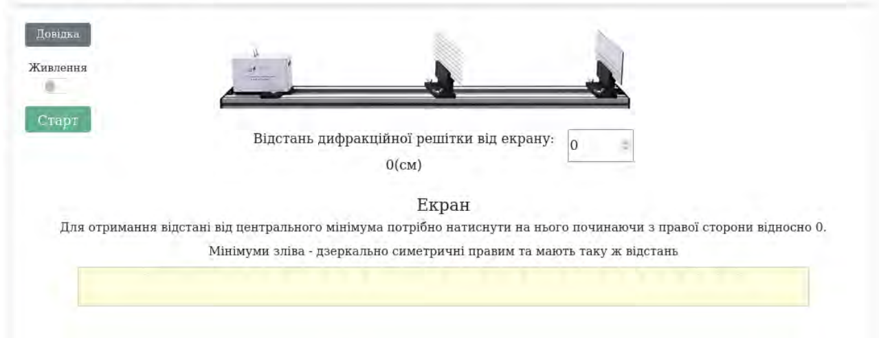
Рисунок 1.13 – Результат розробки емулятора для лабораторної роботи з теми «Вивчення гелій-неонового лазера»
