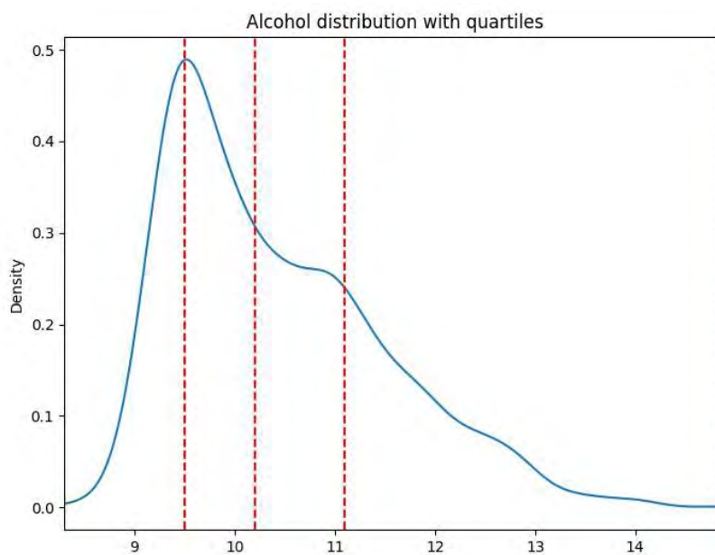
Рисунок 6 – Ілюстрація поділу цільової змінної на категорії
