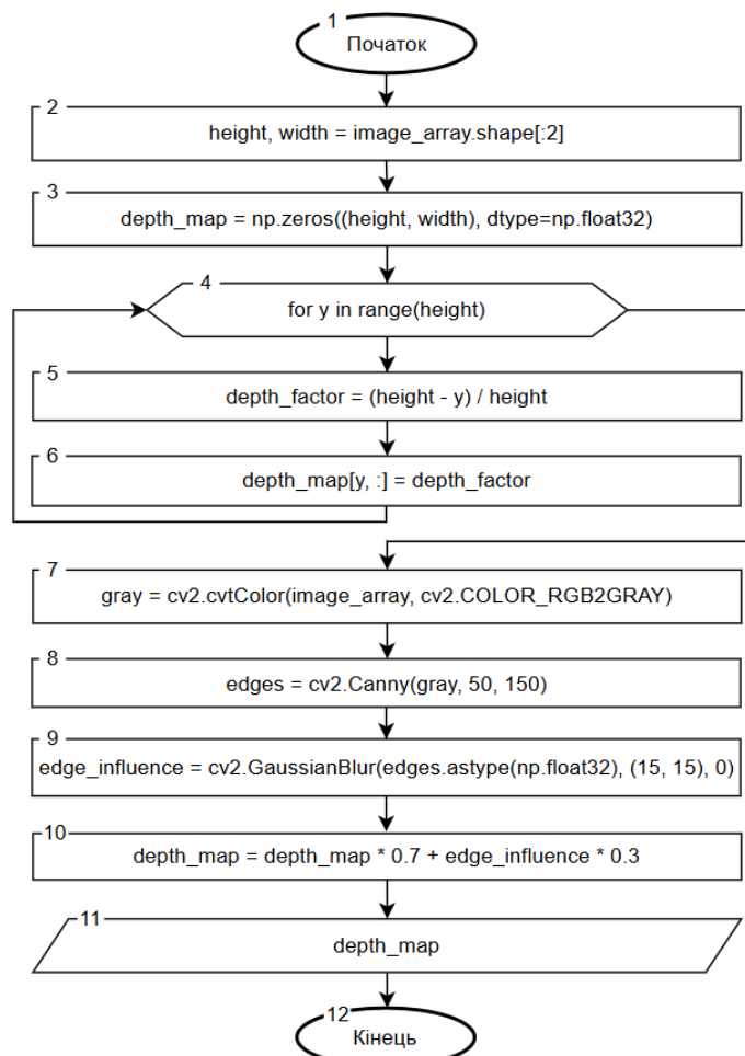
Рисунок 2 - Алгоритм оцінки глибини
