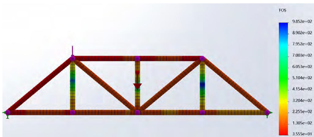
Рис. 4. Епюра розподілу коефіцієнта запасу міцності
