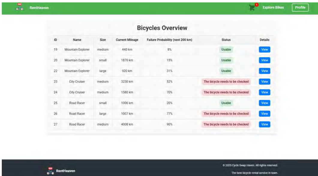
Рисунок 1 – Приклад виведення прогнозування відмови велосипеда
