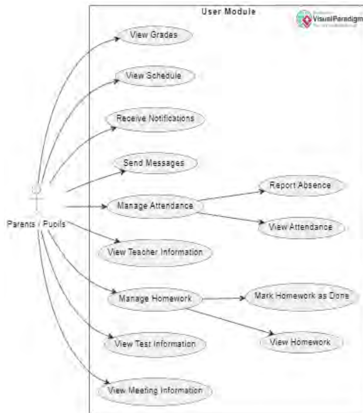
Рисунок 1.2 - Use Case UML-діаграма модуля користувача в ролі Батьки та Учень
