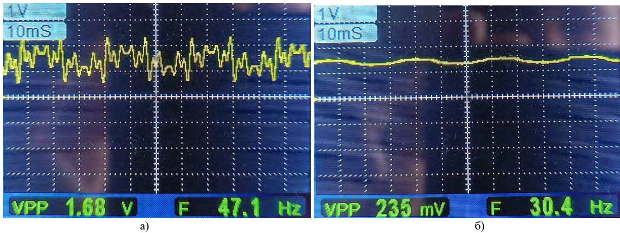
Рис. 1. Діаграма вхідного Signal 1 (a) та Signal 2 (б)
