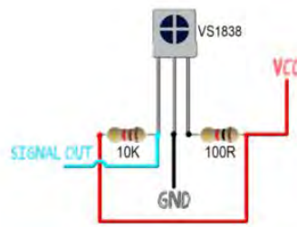
Рисунок 1 - Інфрачервоний приймач VS1838
