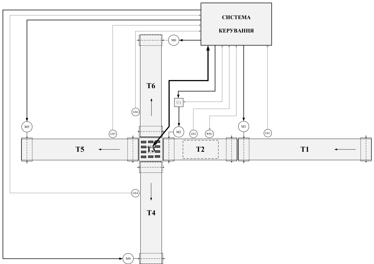
Рис. 1. Схема функціональна системи керування механізмами сортувального відділення
