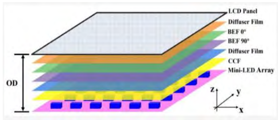
Рисунок 1 – Структура міні-світлодіодної системи освітлення
