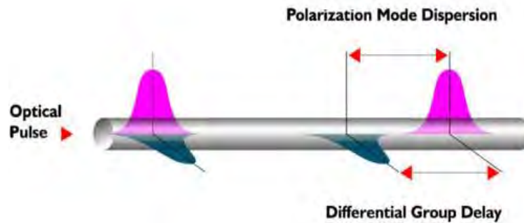
Рис.1 – Схематичне зображення явищ PMD та DGD
