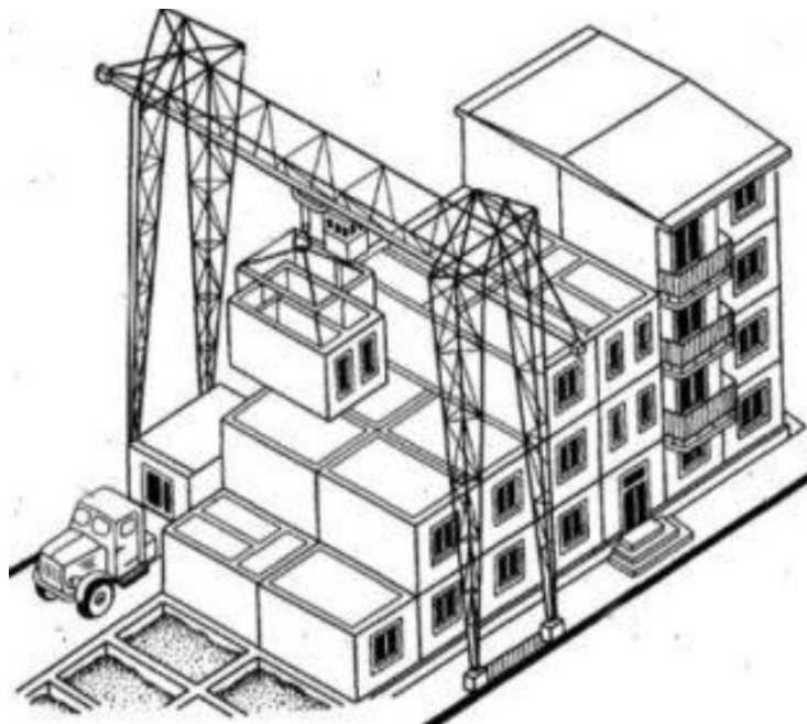
Рисунок 1 – Зведення будівлі з об'ємних блоків
