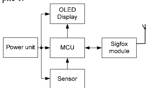
Рис. 1. Структурна схема пристрою моніторингу природного середовища
