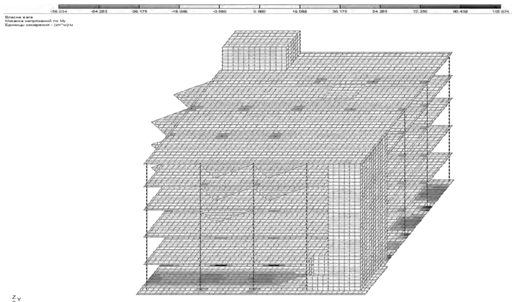
Рисунок 4 – Ізополю внутрішніх зусиль а) M_x , б) M_y скінченно-елементної моделі будівлі в м. Вінниці по вул. Пирогова 89-А
