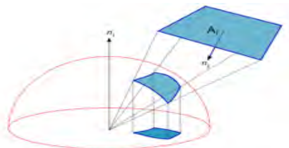
Рис. 3. Проєктування тілесного кута
