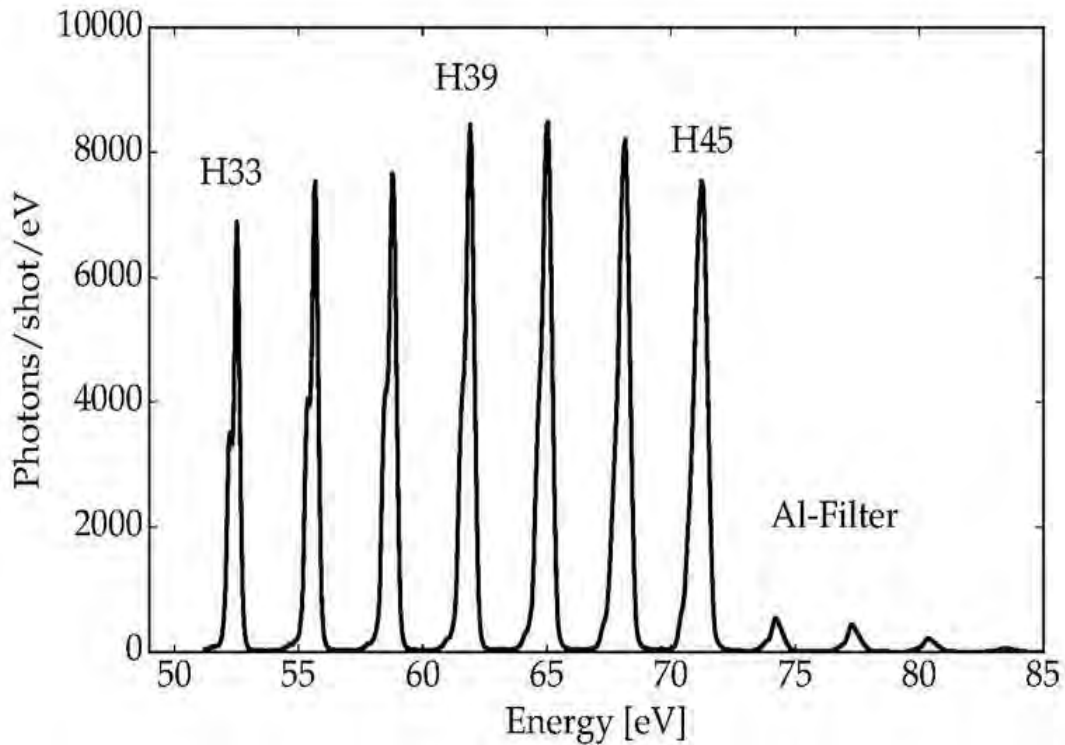
Спектр високих гармонік з плато та зрізом
