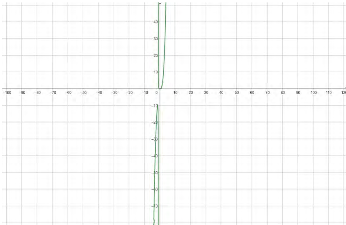
Рис. 1. Графічне представлення розв'язку невизначеного інтеграла
