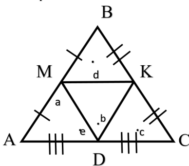
Рисунок 3. – Трикутник ABC з додатково побудованими середніми лініями
