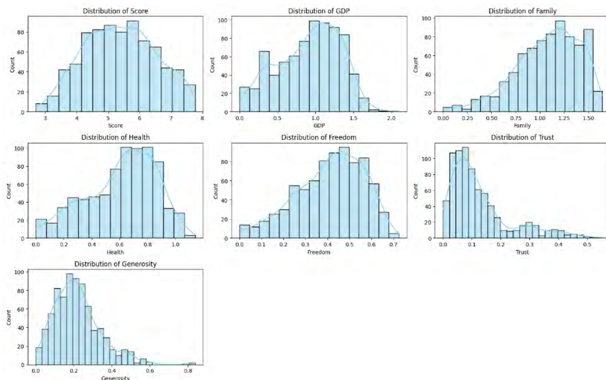
Рис. 2. Гістограма розподілу показників щастя у 2015-2019 роках
