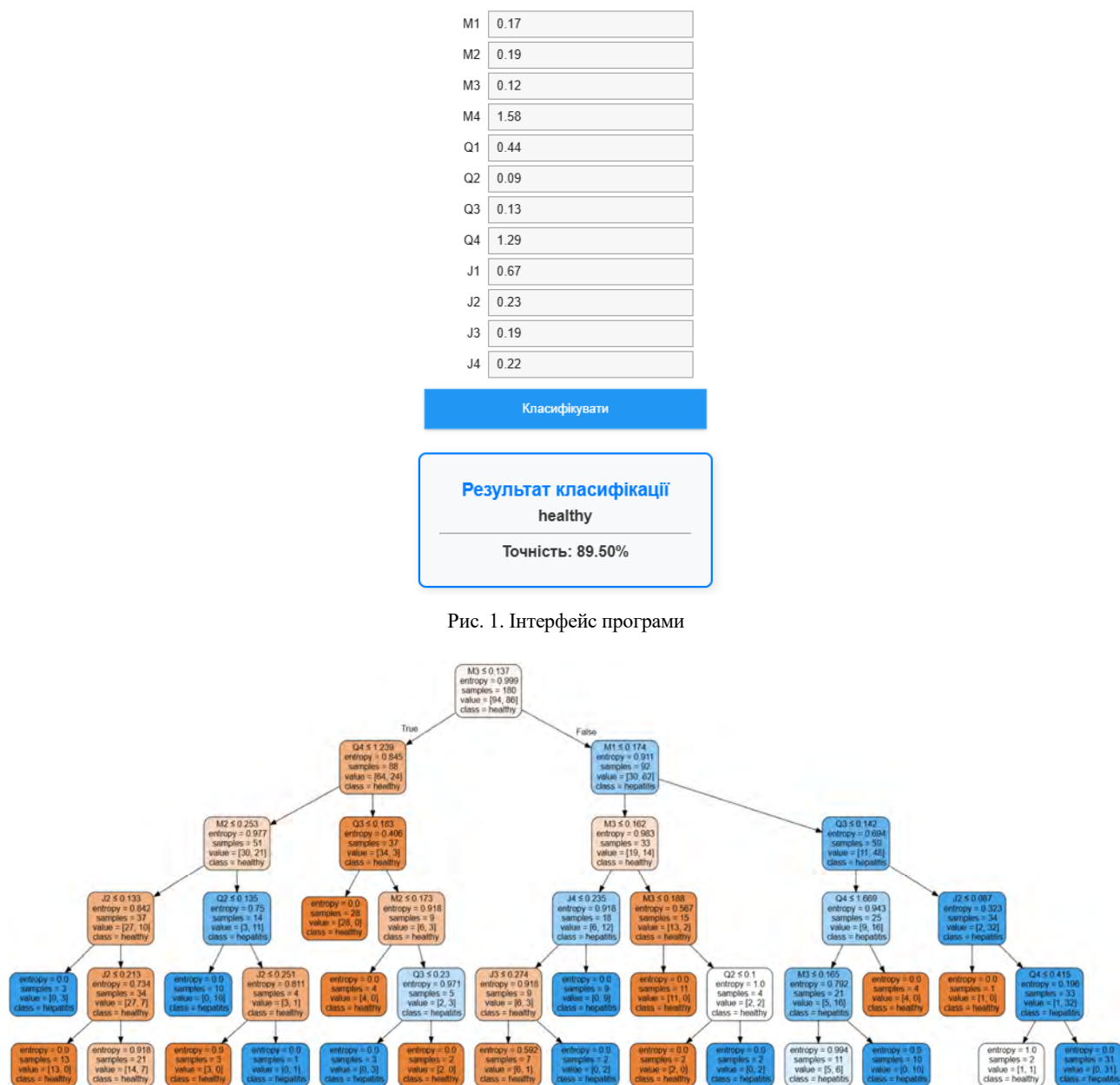
Рис. 2. Візуалізація дерева рішень
