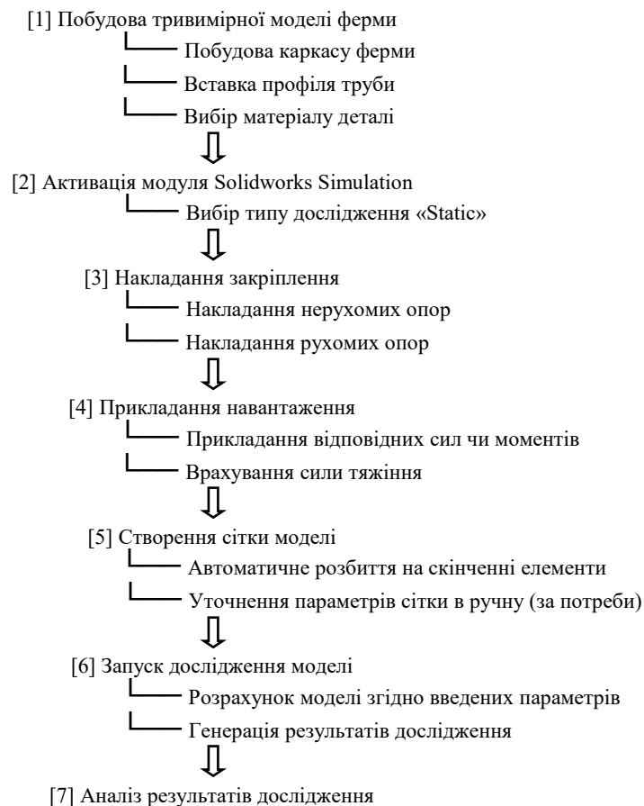
Рис. 1. Алгоритм статичного аналізу зварної конструкції ферми в Solidworks Simulation
