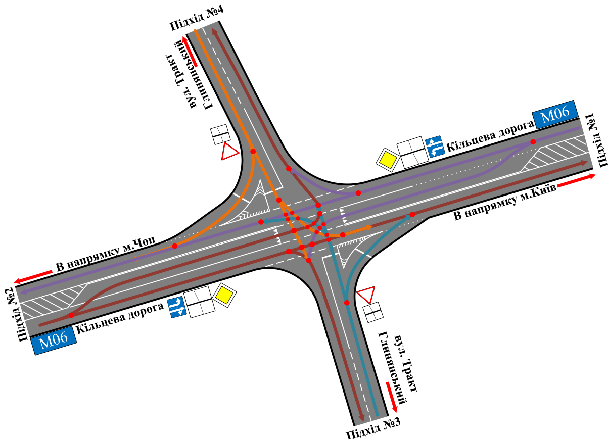
Рисунок 2 – Конфліктні точки на нерегульованому перехресті Кільцева дорога-вул. Тракт Глинянський
