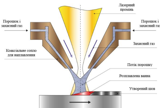
Рис. 7. Лазерне напилення
