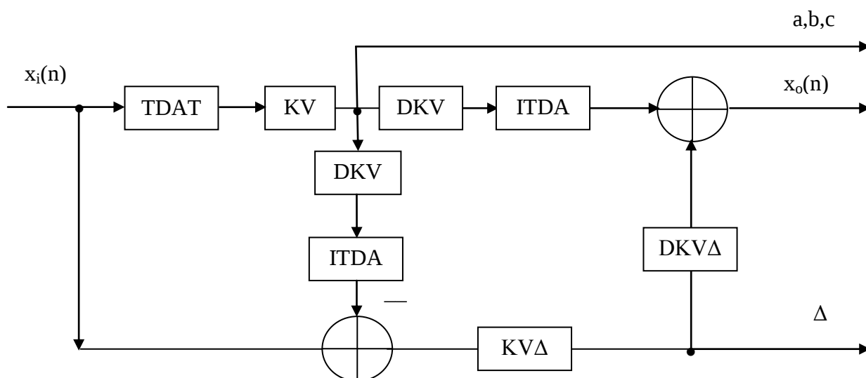
Рисунок 5.1 – Схема ущільнення
