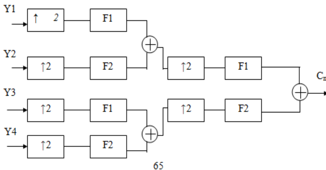
Рисунок 4.3 – Обернене S-перетворення
