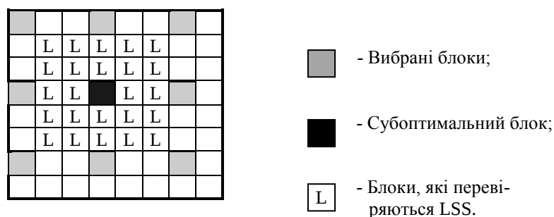
Рисунок 3.5 – Локальний субпошук
