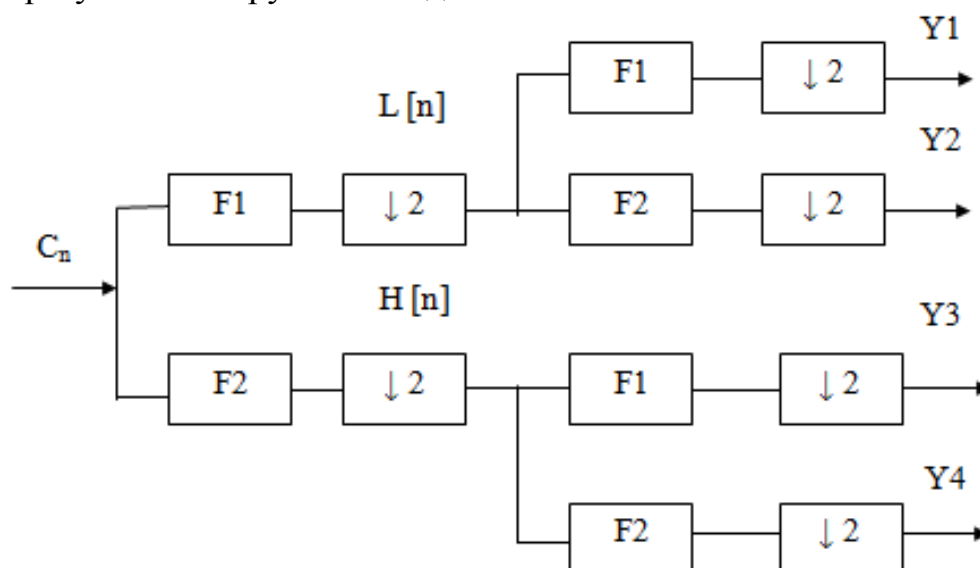
Рисунок 4.2 – Пряме S-перетворення
